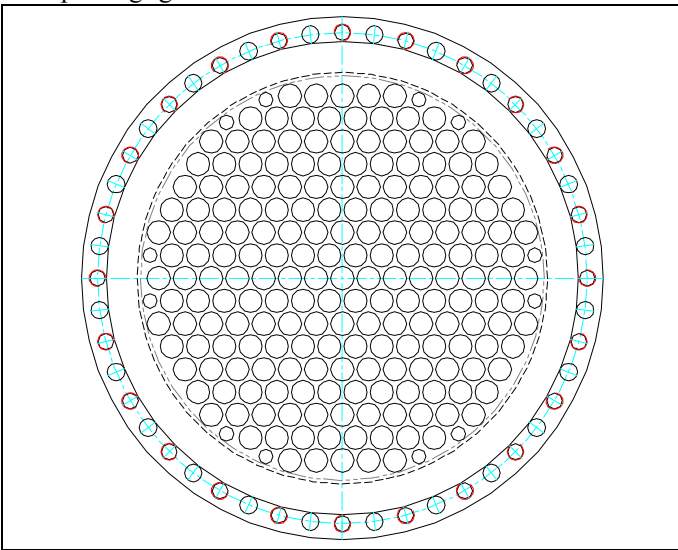
Esempio di griglia
