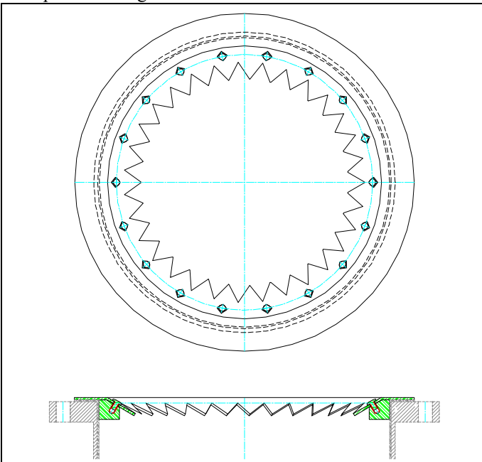
Esempio di convogliatore.
