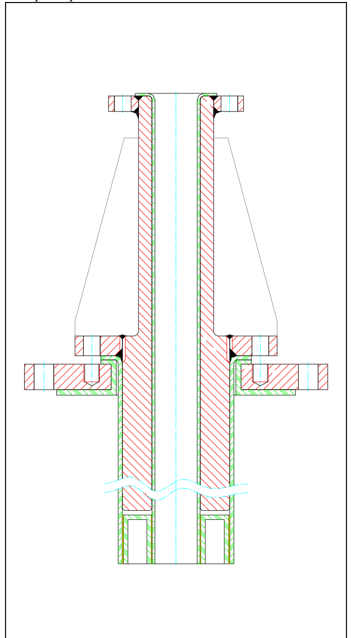
Esempio di pescante ad immersione.
