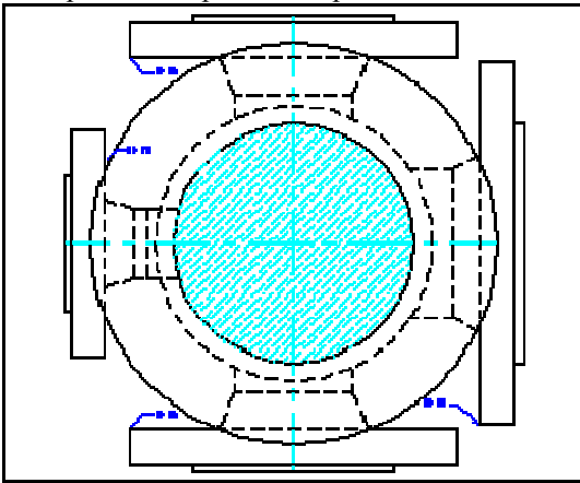
Esempio di una riduzione concentrica speciale.
