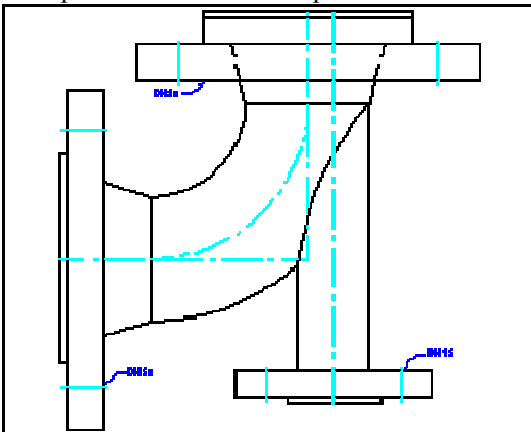
Esempio di una curva a 90° speciale.
